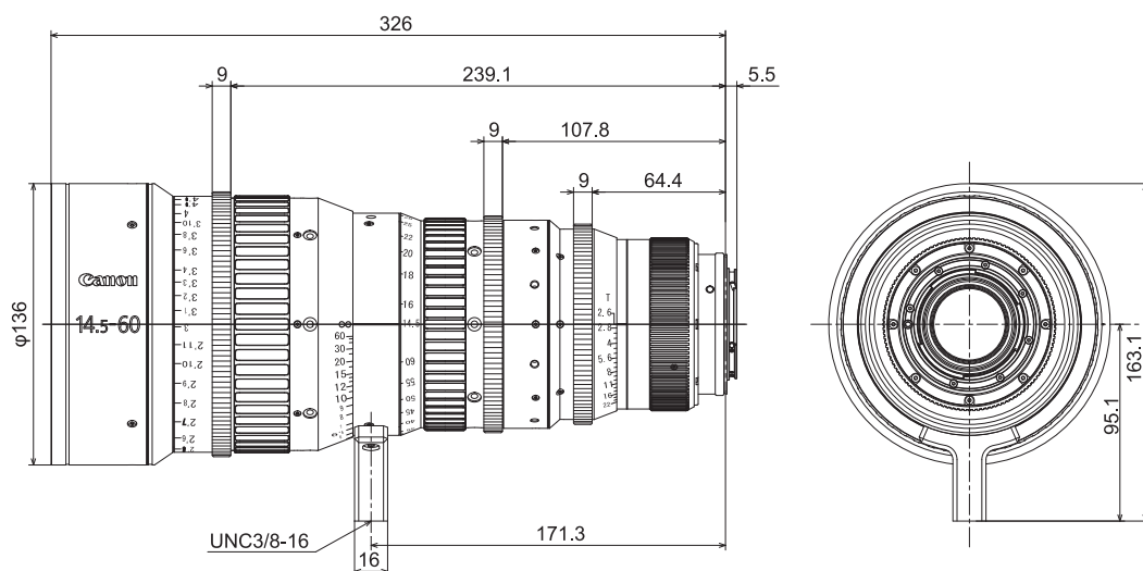
SP型 (PL基座)
