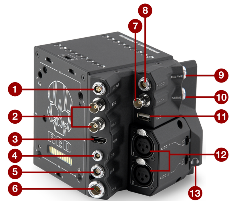
Рисунок Экспандер DSMC2 REDVOLT Expander
