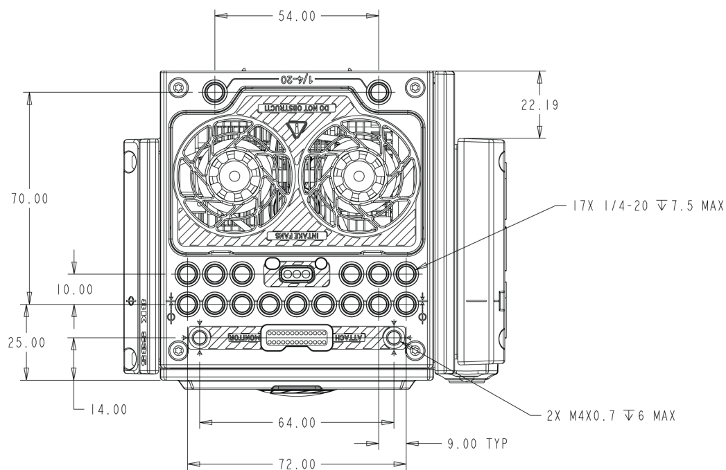
Рисунок Камера EPIC-W, вид сверху
