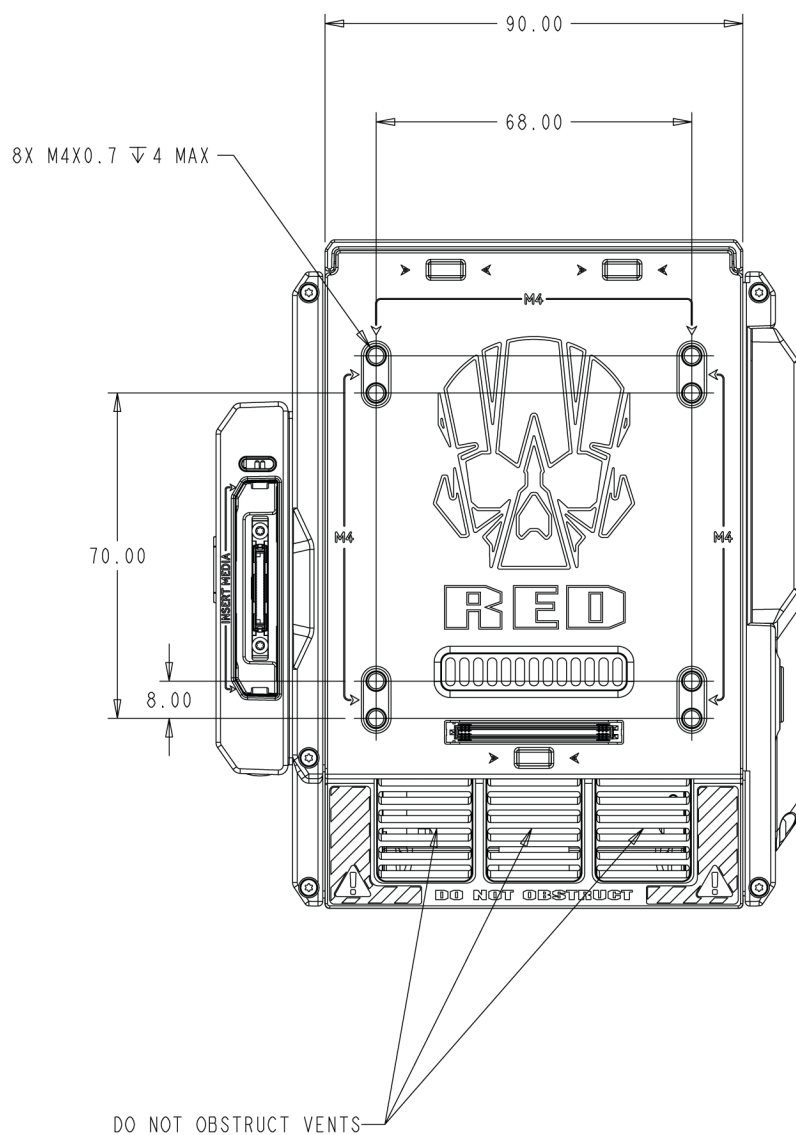
Рисунок Камера EPIC-W, вид сзади
