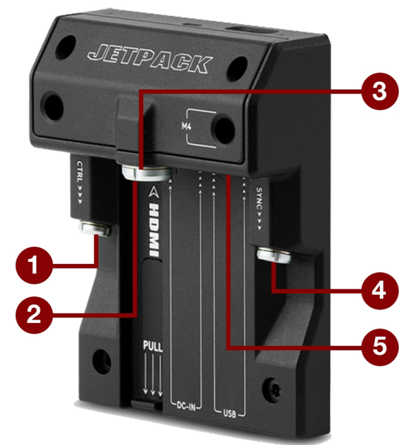
Рисунок Экспандер DSMC2 Jetpack Expander
