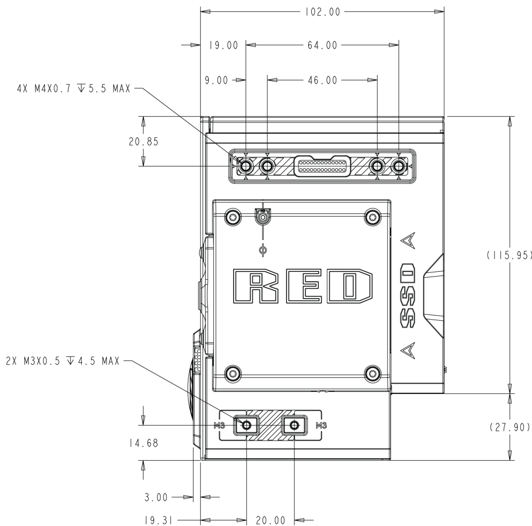
Рисунок Камера WEAPON 8K S35, вид сбоку (справа)
