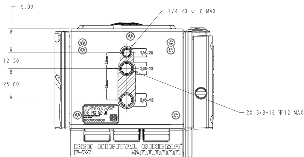
Рисунок Камера EPIC-W, вид снизу
