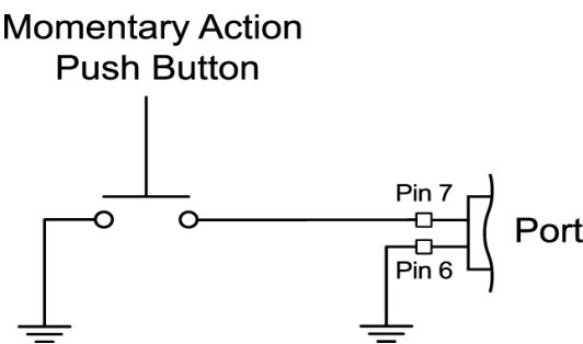
Рисунок Схема цепи кнопки триггера замыкания контактов (SYNC)
