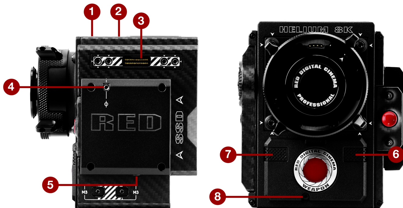
Рисунок Разъемы и функции камеры WEAPON 8K S35 BRAIN
