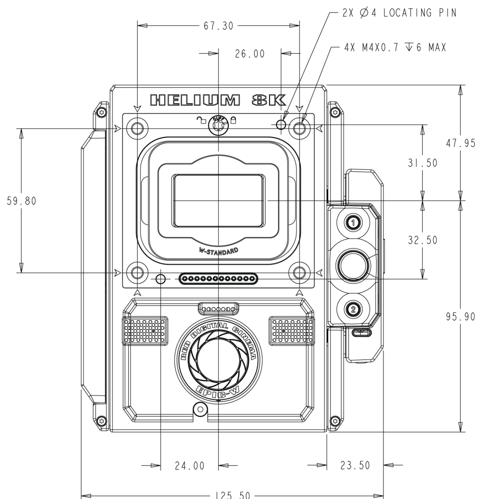
Рисунок Камера EPIC-W, вид спереди
