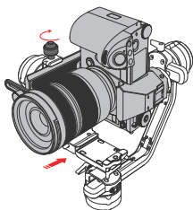
Установка в вертикальном положении
